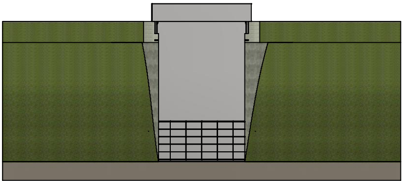
Port lukket (1 : 100)
