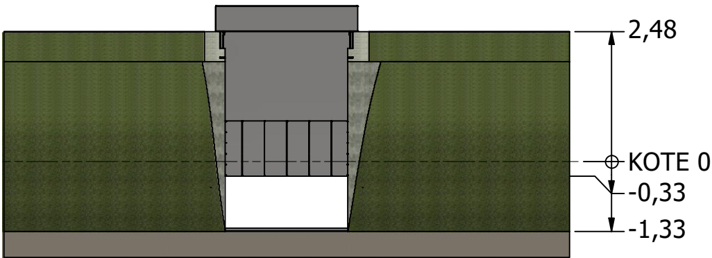
Port åbent ( 1 : 100 )
